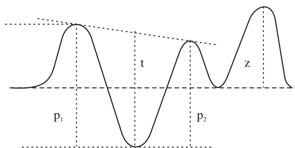
Figura 4. Evaluación de los espectros derivados. Método de la tangente (t), método pico-pico ( p_1 y p_2 ) y método pico-cero (z).
